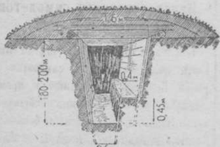
Щель с земляной скамьей, одетой досками.
