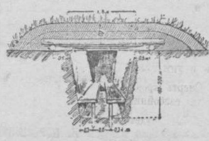
Щель с деревянными скамьями.
