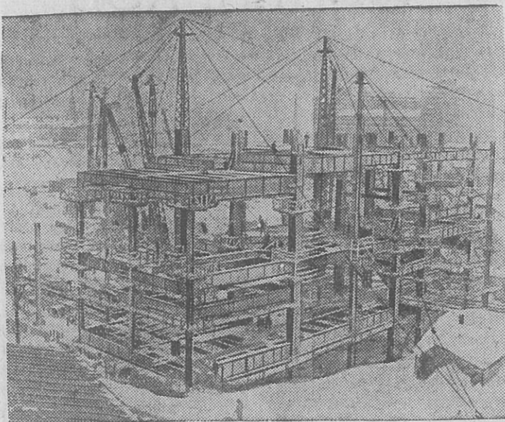
На строительстве Дворца Советов. Первые стальные конструкции металлического каркаса нижней части здания Дворца Советов.
