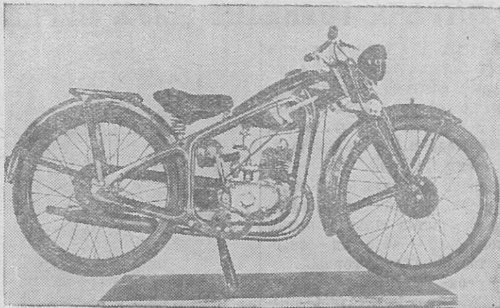
Серпуховский мотоциклетный завод (Московская область) приступил к производству малолитражных мотоциклов «МЛ-3». Вес мотоцикла—70 кг., максимальная скорость 65 км. в час, расход горючего на 100 км. 2½ литра.
