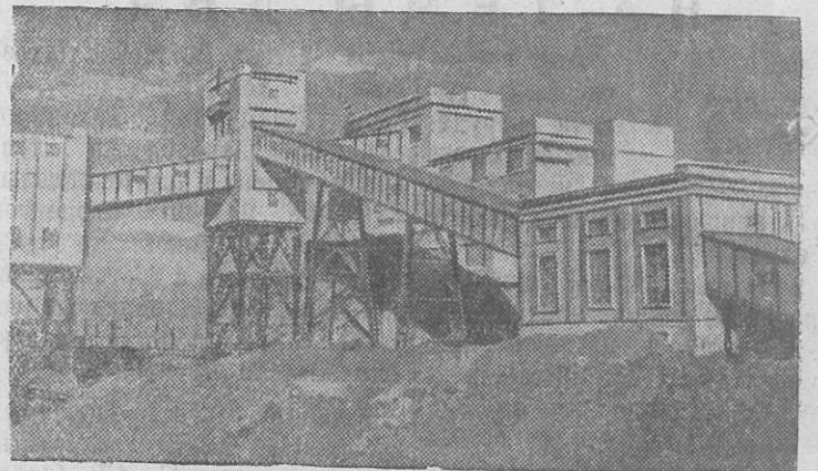
Балхашский медеплавильный завод. НА СНИМКЕ: Корпус среднего дробления и транспортные галереи.
