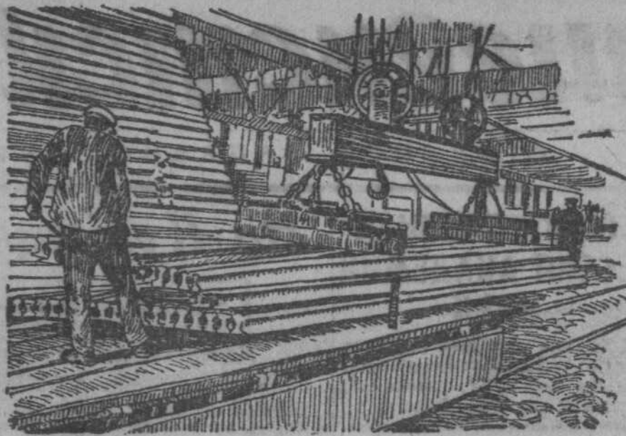
На складе готовой продукции прокатного цеха. На снимке погрузка готовых рельсов в вагоны электромеханическим краном. (Фото Вакнина)
