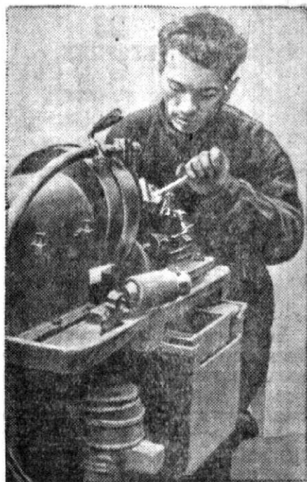
По заданию наркома тяжелой промышленности Ленинградский завод им. Ильича изготовил станок для заточки буровых коронок. Подобных станков заграницы еще нет. На снимке: слесарь-оборщик В. М. Никаноров проверяет новый станок. СЮЗФОТО.
