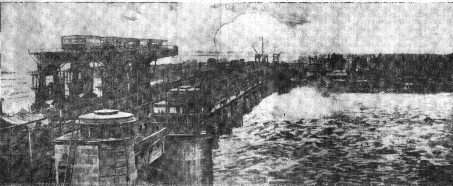
КАНАЛ ВОЛГА—МОСКВА. На снимке: общий вид Верхневолжской плотины.
