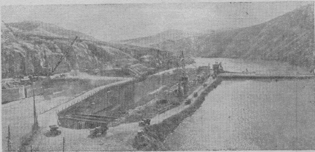
Восточно-Казахстанская область. Строители Бухтарминской ГЭС одержали большую трудовую победу. Досрочно затоплен котлован первой очереди и перекрыт Иртыш. На снимке: общий вид стройки со стороны нижнего бьефа.
