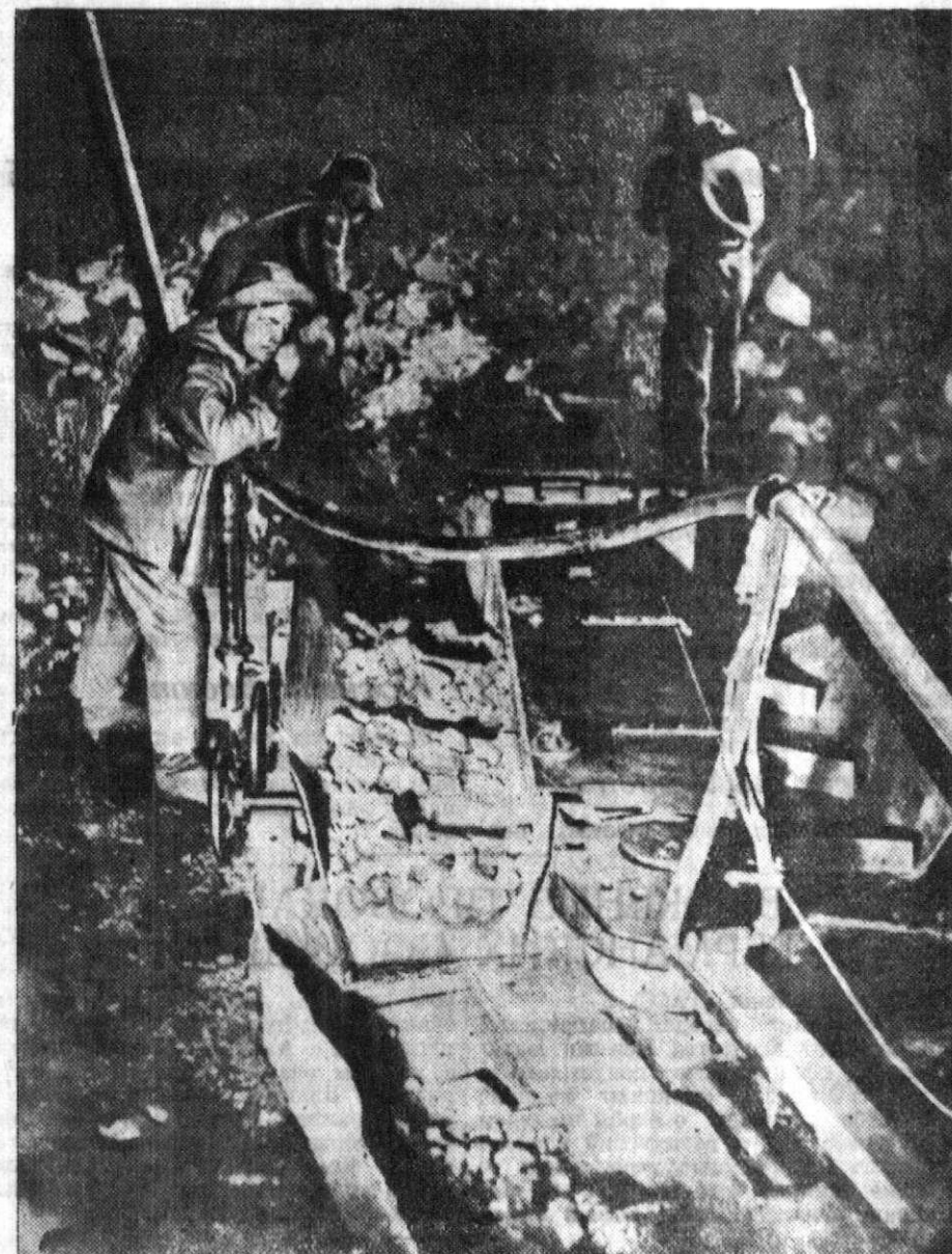
Тяжелая врубовая машина «Шортленд» в шахте (Прокопьевск). Фото Н. МЕЛНХОВА.
