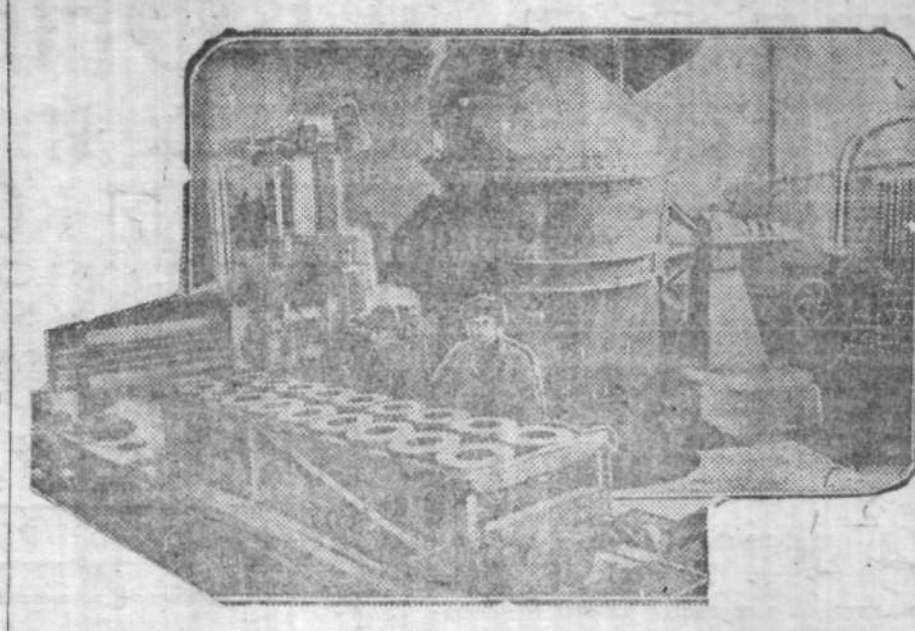
Овладевая техникой! рабочие и специалисты литейного цеха Шагского химзавода, своими силами изготовили конвейер системы «Робера» для фосоного литья, вместимостью 1 тонна.
