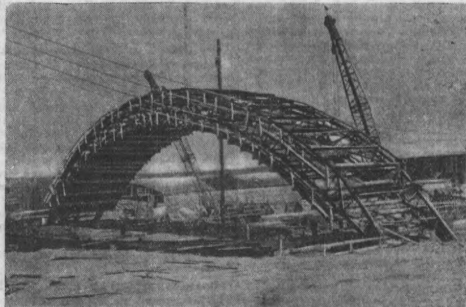
На строительстве Куйбышевского гидроузла. На снимке: общий вид монтажа металлического перекрытия гидротехнической лаборатории. Фотографии ТАСС
