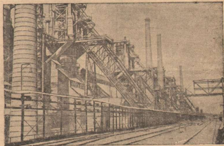
Вид на один из уголков доменного цеха Кузнецкого металлургического комбината имени Сталина.
