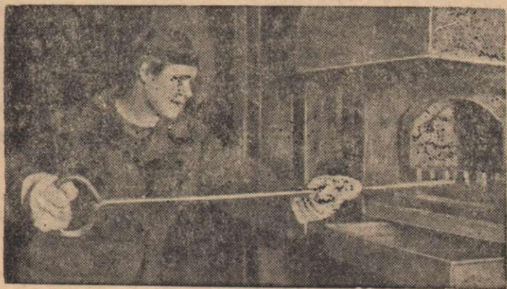
Бригадир женской бригады обжига молибденового концентрата Челябинского ферросплавного завода имени Ворошилова, комсомолка Х. И. Кулакова наблюдает за ходом обжига концентрата. Фото В. Тишечкина.
