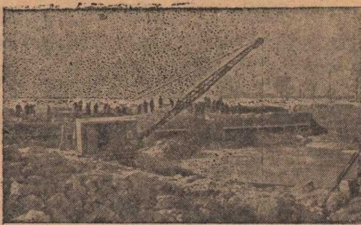
В Западных областях Белоруссии идет строительство Днепро-Бугского канала протяжением в 202 километра. Канал соединит судходную реку Буг с Днепром и Черным морем. Строительство канала предполагается закончить в апреле тек. года. На снимке: На строительстве 10-го гидроузла Днепро-Бугского канала
